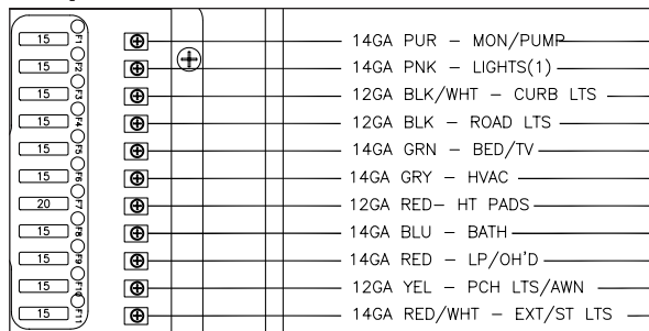
30 Amp DC circuits
