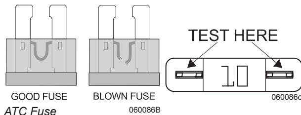
ATC Fuse
