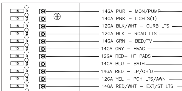
50 Amp DC circuits
