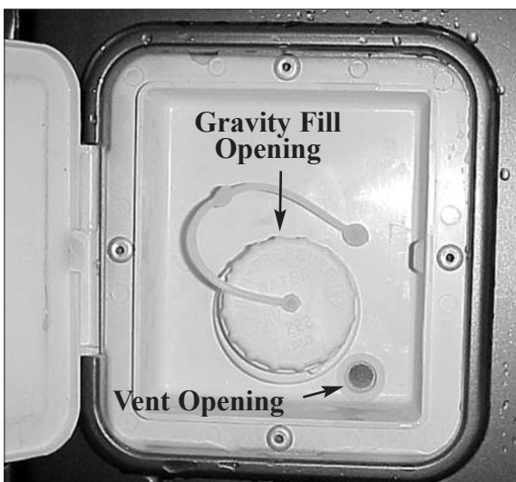
Gravity Fill Tank.
